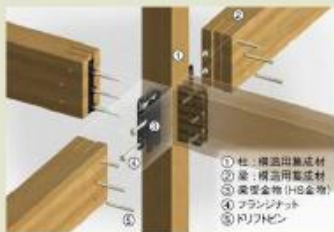
構造材を強固に接合する「スペースロック工法」
